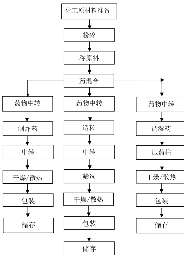
图 2.3-2 药物裸药效果件（炸药、亮珠、药柱）生产工艺流程图
