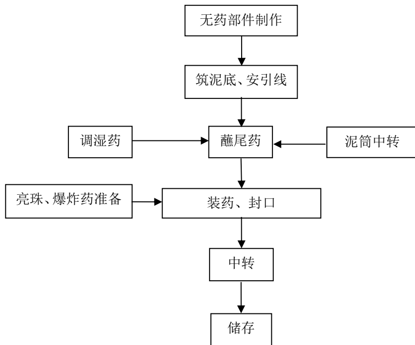
图 2.3-1 效果件内筒生产工艺流程图
