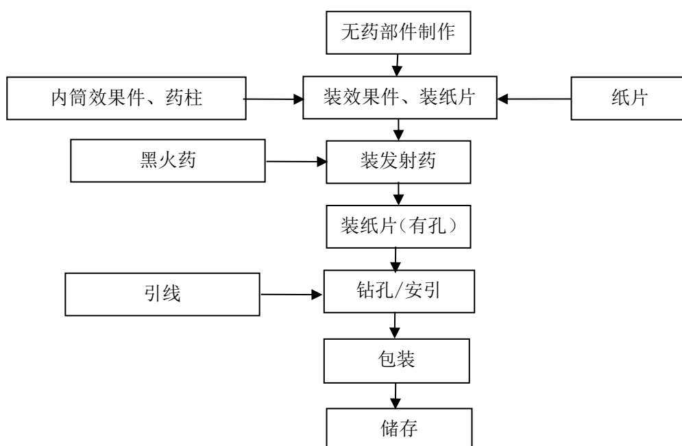
图 2.3-5 礼花类（小礼花/柱形）产品生产工艺流程图
