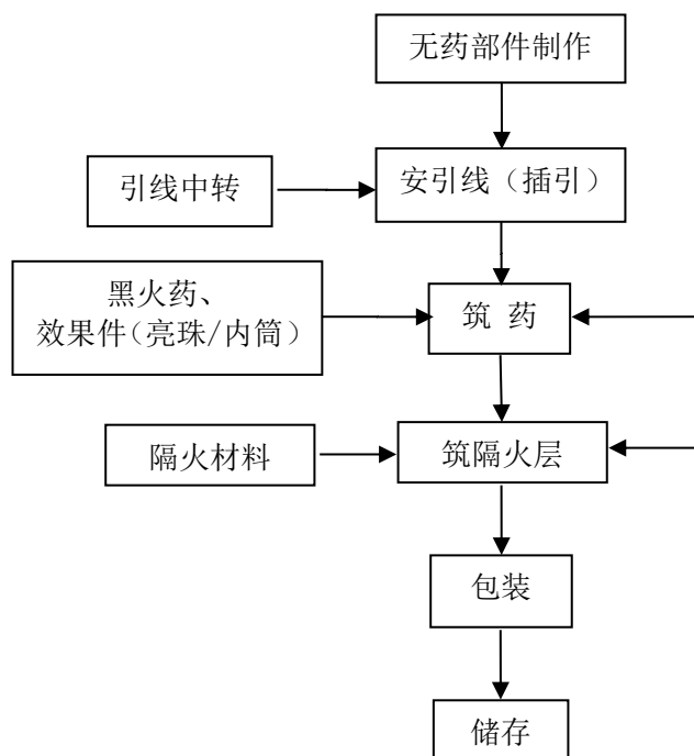
图 2.3-5 礼花类（小礼花/柱形）产品生产工艺流程图
